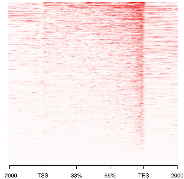
GMtr_0h_CHIPSeq_untr_medium
