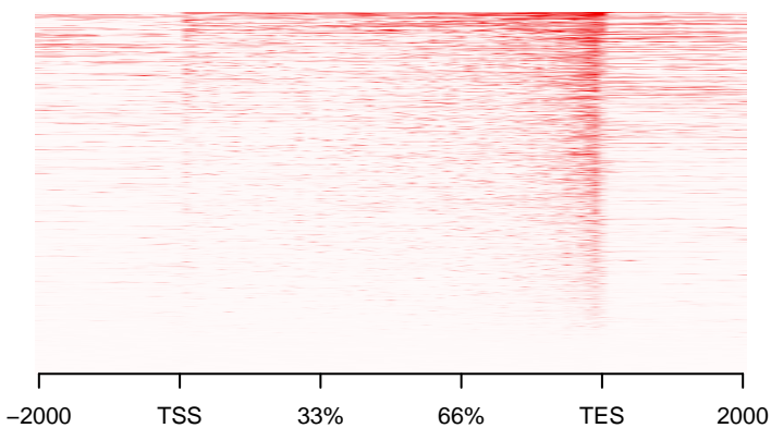
GM_untr_CHIPSeq_untr_low
