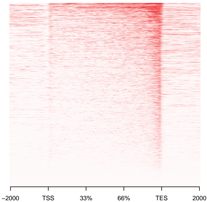
GM_untr_CHIPSeq_untr_medium
